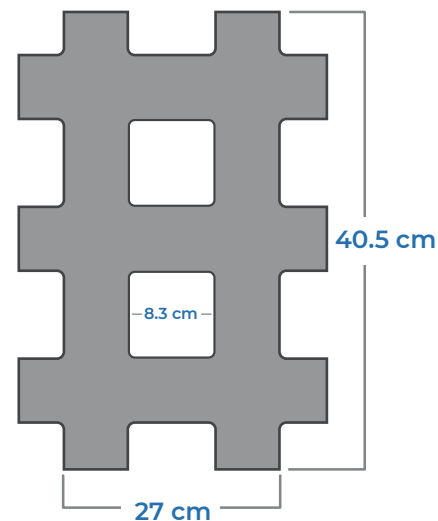
Vista inferior
